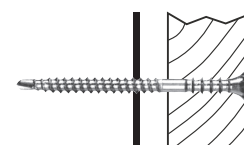
Infästning i ståltjocklek upp till max 1,2 mm, dras direkt utan förborring.
